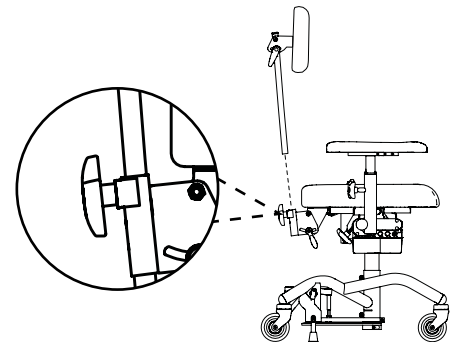
Figuur 5.7. Rugsteunmechanisme Standaard röntgen.
