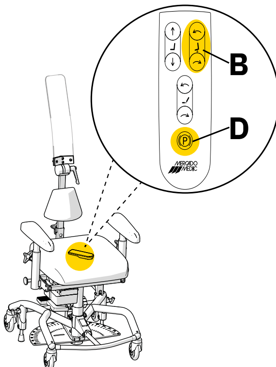
Figuur 2.3. Bedieningselementen van de REAL 8100 PLUS 24V Advanced.
