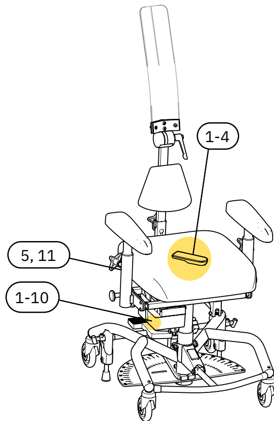
Figuur 7.1. Overzicht van symbolen op bedieningselementen op het product.
