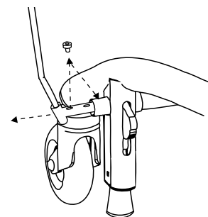
Figuur 5.20. Instelling van remhendelbeugel.
