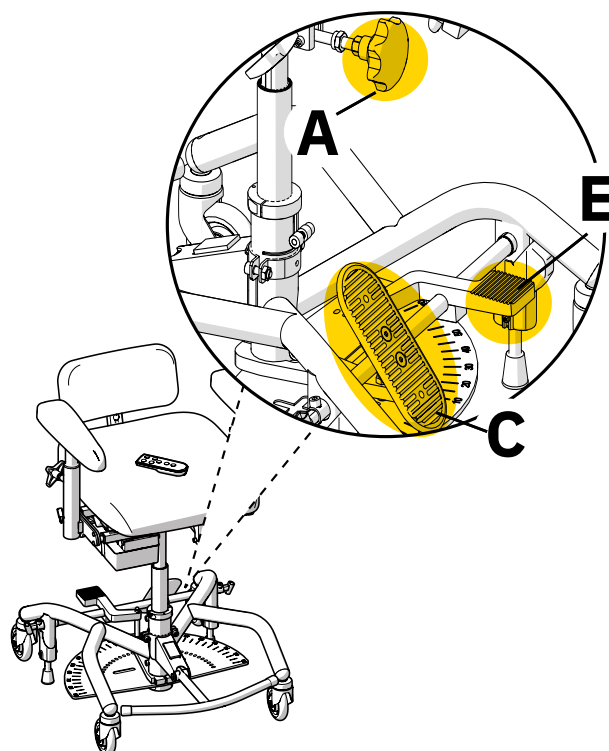
Figuur 2.2. Bedieningselementen van de REAL 8100 PLUS 24V Standaard.
