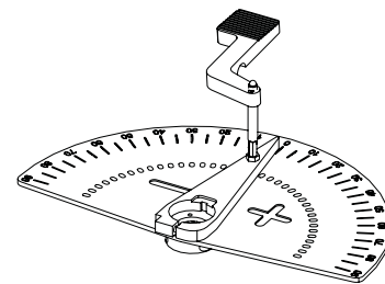
Figuur 5.16. Gradenschijf met rotatievergrendeling.
