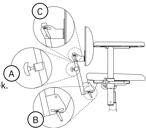
Figuur 5.8. Rugsteun ErgoMedic.
