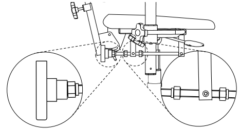
Figuur 5.6.1. Zwengel voor het instellen van de zittingkanteling.
