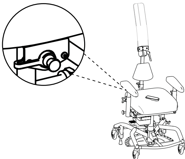
Figuur 2.4. Sluit de stekker aan op het laadcontact onder de zitting.
