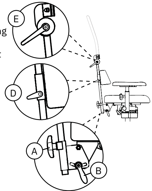
Figuur 5.9. Hoge rug met verstelbaar kussen en hoofdsteun van Macrolon.
