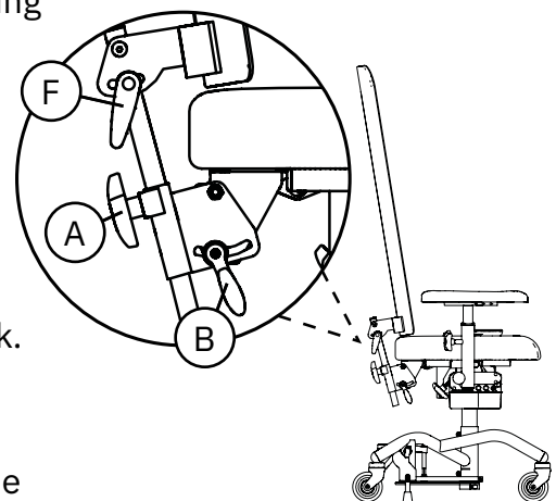
Figuur 5.10. Hoge transparante rugsteun.
