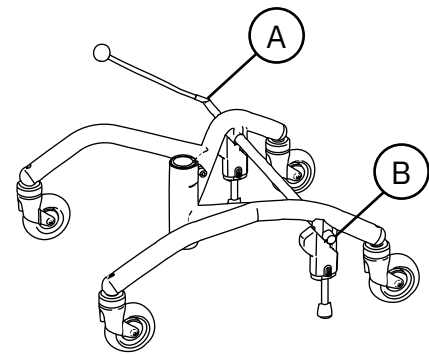
Figuur 5.19. Remhendel.
