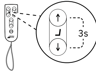
Figuur 5.4. Activeren en deactiveren van toetsvergrendeling.
