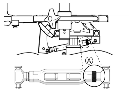
Abb. 5.6.1. Drehspindel zur Einstellung des Sitzwinkels.
