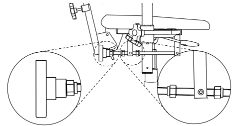
Abb. 5.6.1. Drehspindel zur Einstellung des Sitzwinkels.
