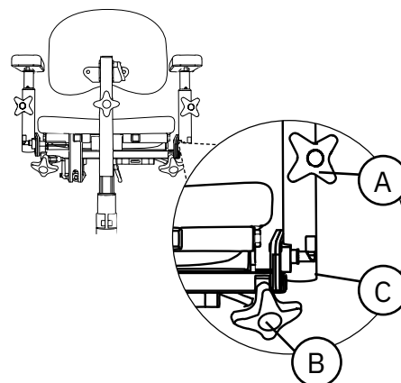
Figur 5.14. Fällbara armstöd.
