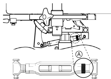
Figur 5.6.2. Vantskravsreglage för justering av sitstilt.
