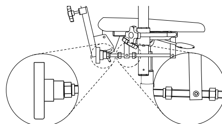
Figur 5.6.1. Vevreglage för justering av sitstilt.
