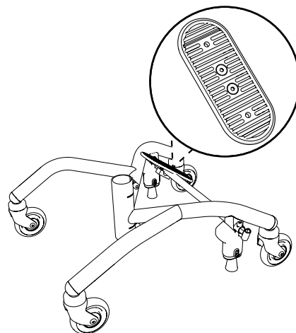
Figur 5.18. Fotbroms.
