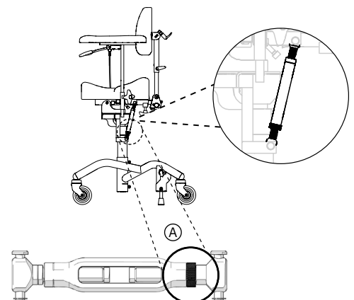
Abb. 5.19. Drehspindel zur Einstellung des Sitzwinkels.
