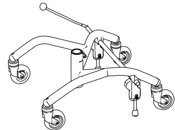
Abb. 5.35. 9000 PLUS-Rahmen 48.
