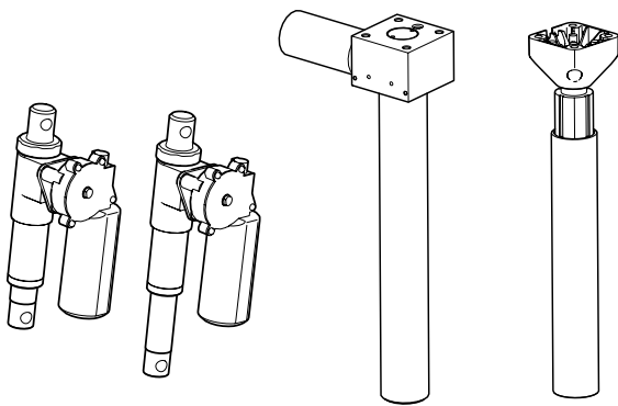
Abb. 3.1. Hubvorrichtung und sonstige Stellantriebe des Produkts.
