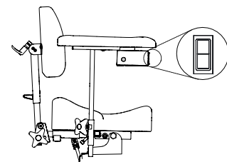
Abb. 5.1. Schalter zur Einstellung der Sitzhöhe.
