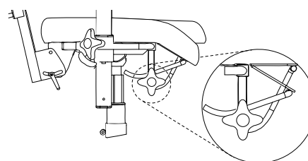
Figure 5.33. Réglage sous le bord avant de l'assise permettant d'ajuster le mécanisme Coxit.
