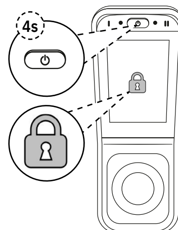
Figure 5.13. Verrouillage des boutons sur LiNX REM400.
