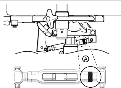
Figure 5.32.1. Réglage par manivelle pour ajuster l'inclinaison de l'assise.
