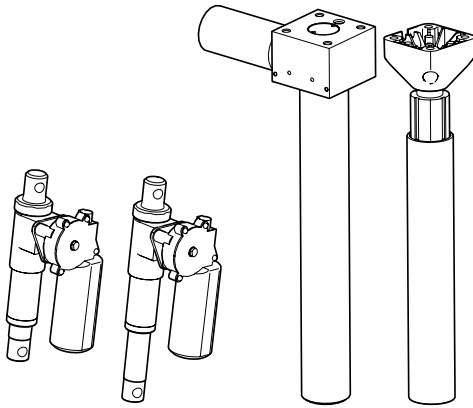
Figure 3.1. Élévateur du produit et autres actionneurs.
