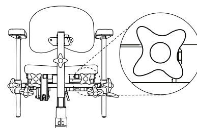
Figure 5.34. Réglage sous le bord arrière de l'assise permettant d'ajuster le mécanisme Coxit.
