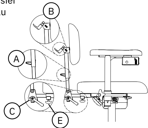
Figure 5.42. Mécanisme de dossier Medic.
