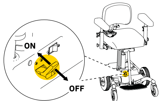
Abb. 3.2. Entkuppelung der Bremse.
