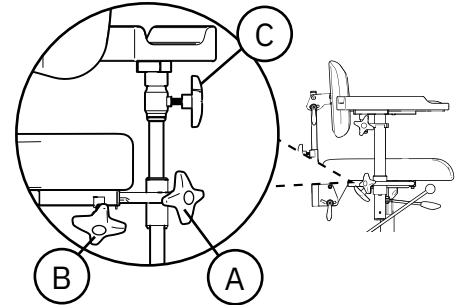
Abb. 5.51. Hemiplegie-Armlehnen.
