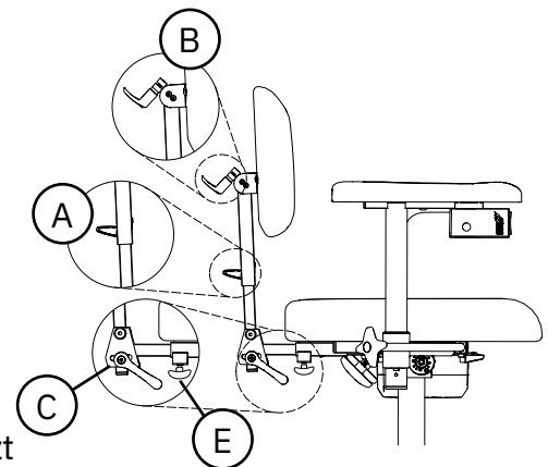
Abb. 5.42. Rückenlehnenmechanismus Medic.
