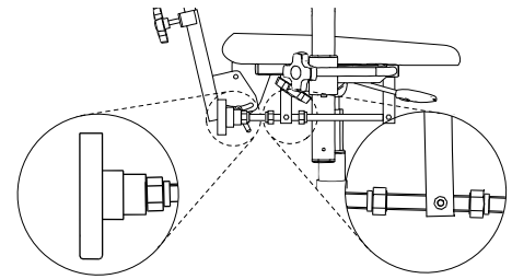
Abb. 5.32.1. Drehspindel zur Einstellung des Sitzwinkels.
