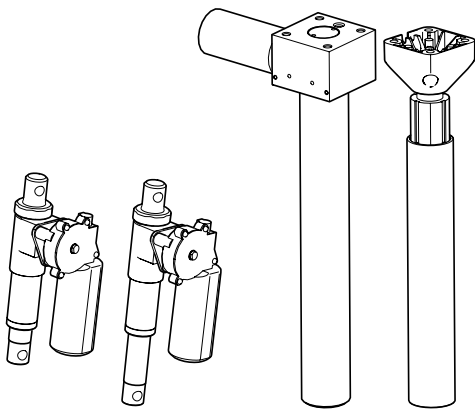
Abb. 3.1. Hubvorrichtung und sonstige Stellantriebe des Produkts.
