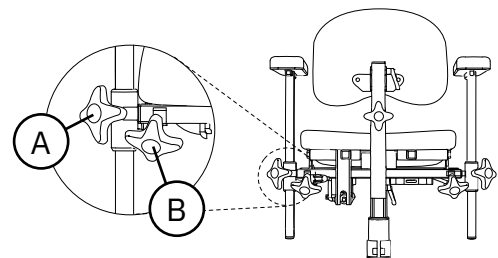
Abb. 5.50. PLUS-Armlehnen.
