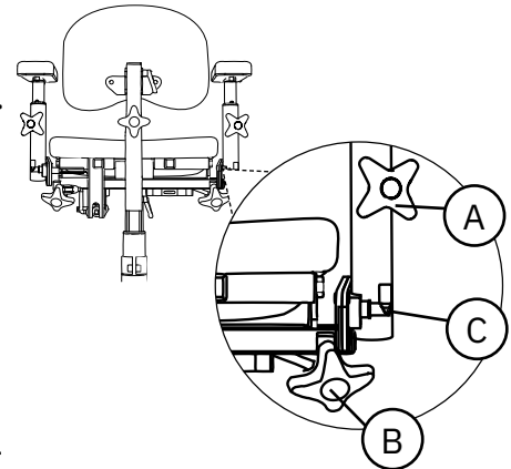
Abb. 5.49. Wegklappbare Armlehnen.
