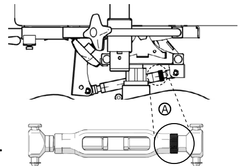
Abb. 5.32.2. Spannschloss zur Einstellung der Sitzwinkels.
