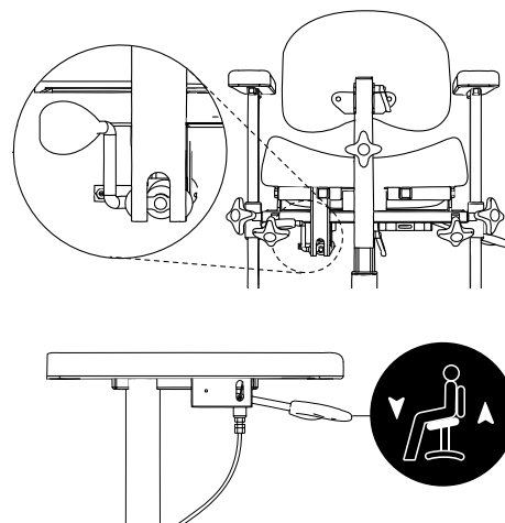
Figur 5.31. Gasfjäderreglage för justering av sitstilt.
