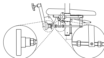
Figur 5.32.1. Vevreglage för justering av sitstilt.
