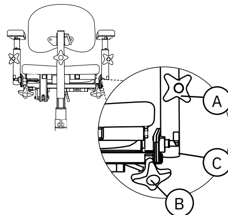
Figur 5.49. Fällbara armstöd.
