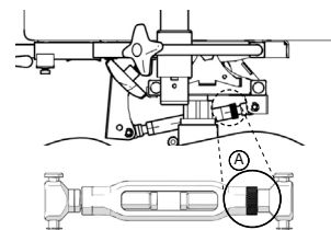
Figur 5.32.2. Vantskravsreglage för justering av sitstilt.
