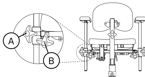
Figur 5.50. PLUS-armstöd.
