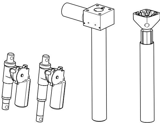
Abb. 3.1. Hubvorrichtungen und sonstige Stellantriebe des Produkts.
