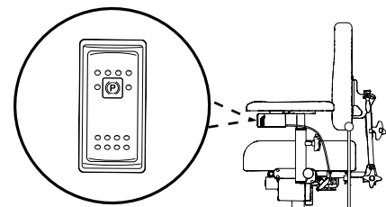
Abb. 5.2. Schalter zum Aktivieren und Deaktivieren der Bremse.
