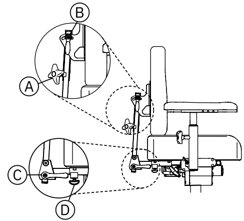
Abb. 5.9. Rückenlehnenmechanismus Medic TWIN.
