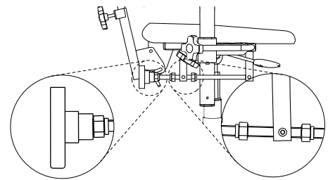
Figuur 5.16.1. Zwengel voor het instellen van de zittingkanteling.
