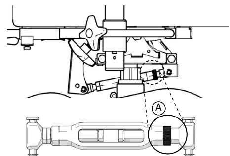
Figuur 5.16.2. Spanschroef voor het instellen van de zittingkanteling.
