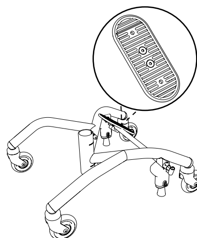
Figur 5.49. Fotbroms.
