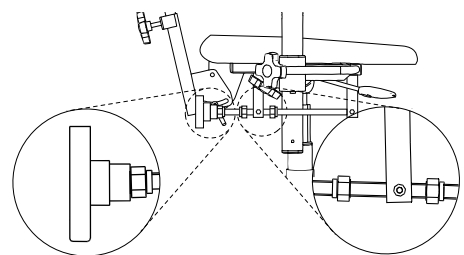
Figur 5.16.1. Vevreglage för justering av sitstilt.
