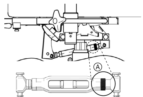
Figur 5.16.2. Vantskravsreglage för justering av sitstilt.
