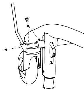
Figur 5.48. Inställning av bromsspaksfäste.
