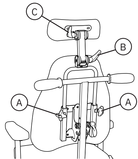
Afbeelding 5.10. Hoofdsteen
