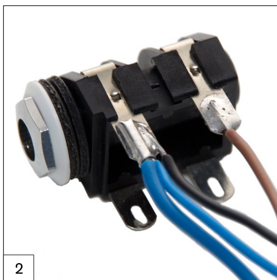
Bild [2] visar laddjacket som det är kopplat från v. 11 2013, där de blå kablarna sitter på samma sida som den svarta minuskabeln. Denna koppling tar bort problemet med att kortet tror att stolen laddas och därför inte kan köras.
